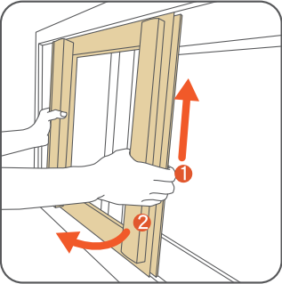
拆卸大鉤扇：雙手緊握大鉤扇窗緣，1 向上提起，2 下方朝內即可卸下
