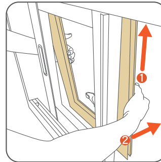
拆卸紗窗扇：雙手在室內向外緊握窗緣兩旁，1 向上提起，2 下方朝外推出卸下
