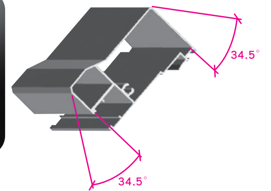
內門橫料 | 鑽石切割 |
