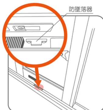
拆卸小鉤扇：拉至將防墜落器對準中間排水口，雙手緊握窗緣兩旁向上提起，下方朝外推出卸下
