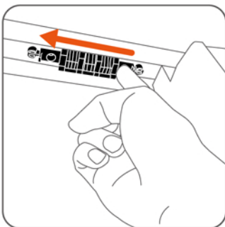
將上阻風板拉出(解除大鉤扇防落)
